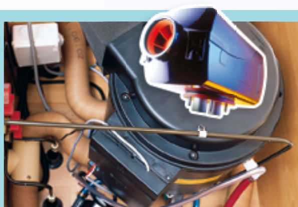
La chaleur ambiante est assurée grâce à un chauffage à air pulsé utilisant le carburant du véhicule ou le gaz (utilisable en roulant)*.
