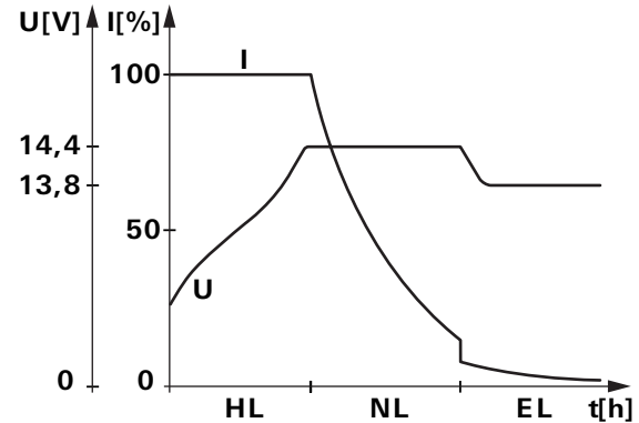
Bild 2: Ladekennlinie (princieller Verlauf)
